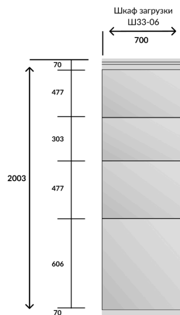
Шкаф загрузки с одной ячейкой выдачи
